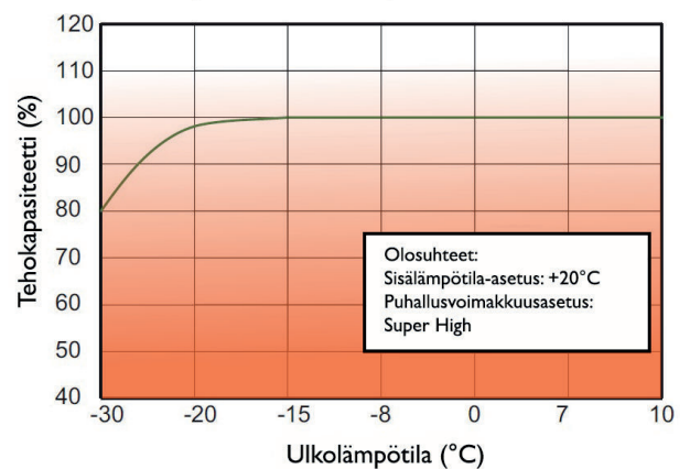
Lämmitysteho eri ulkolämpötiloissa
